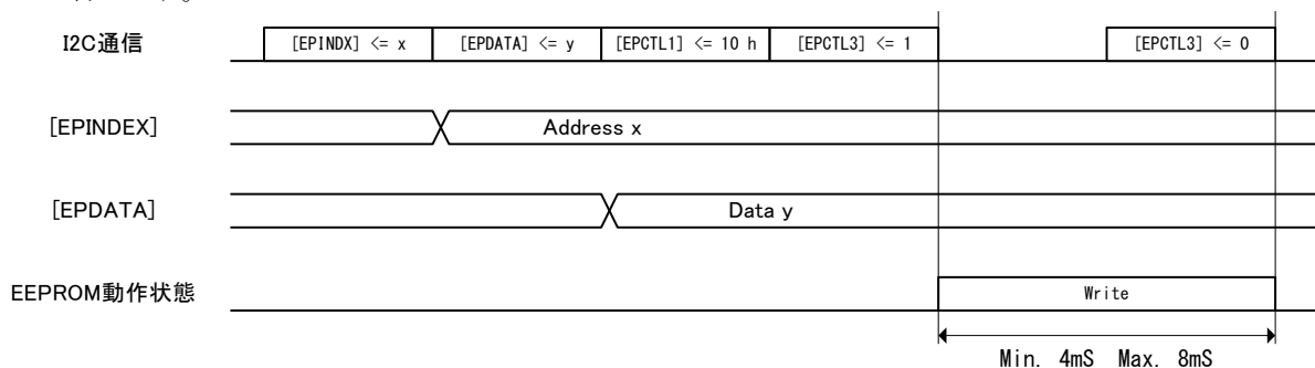
図 8-6 ブロック書き込み動作
