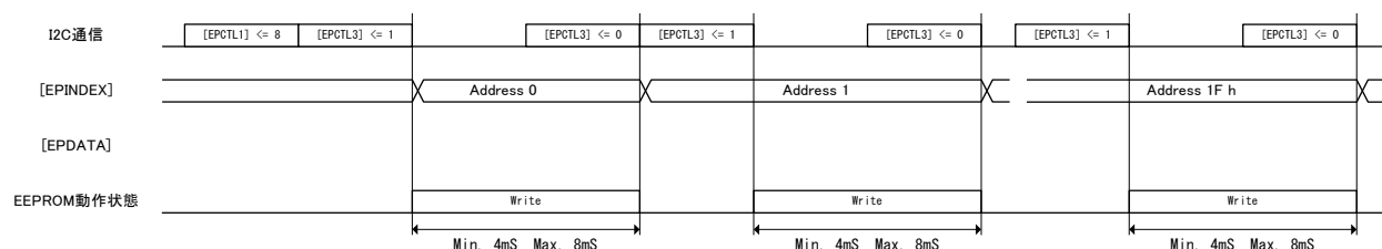
図 8-4 ブロック書き込みシーケンス
