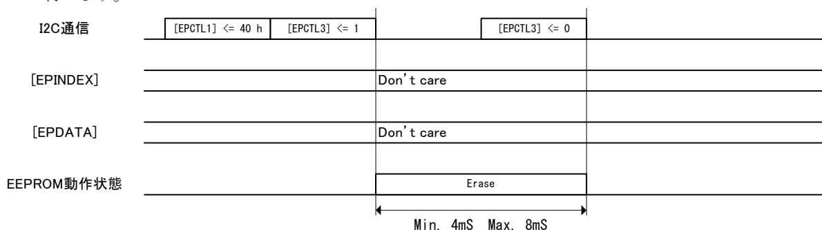
図 8-5 ブロック消去動作
