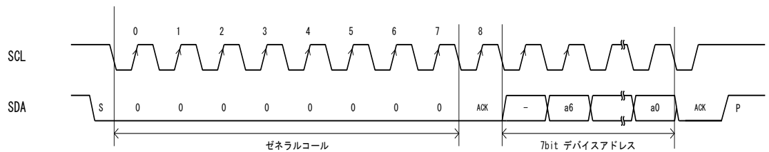
デバイスアドレス設定タイミング
